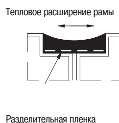
Рис. 5 Расположение разделительного жгута пленки для предотвращения крепления уплотнителя к трем поверхностям
