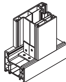
Узел в сборе
