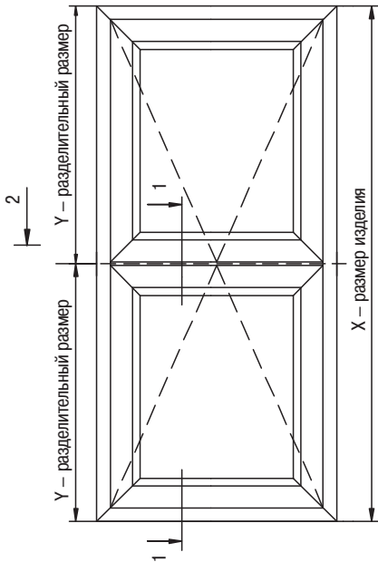
Двустворчатое окно (со штульпом). Вид «А»
