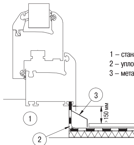
Рис. 10. Примыкание балконной двери к покрытию террасы.
