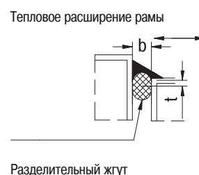
Рис. 5 Расположение разделительного жгута пленки для предотвращения крепления уплотнителя к трем поверхностям
