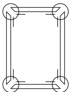
Сварной соединитель дверных углов «27х35» в сборе (корпус, клин, винт)
