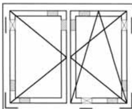
Двустворчатое окно с поворотной и поворотной-откидной створкой.
