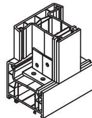
Узел в сборе
