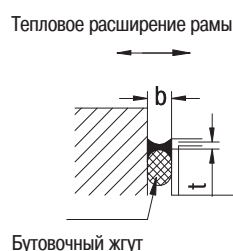
Рис. 3 Разрез по плоскости уплотнения (нагрузка сжатия и растяжения)
